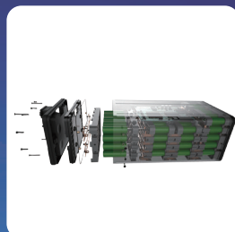
Batterie lithium polymère à 3 parties GREENWAY 48V - 26Ah
